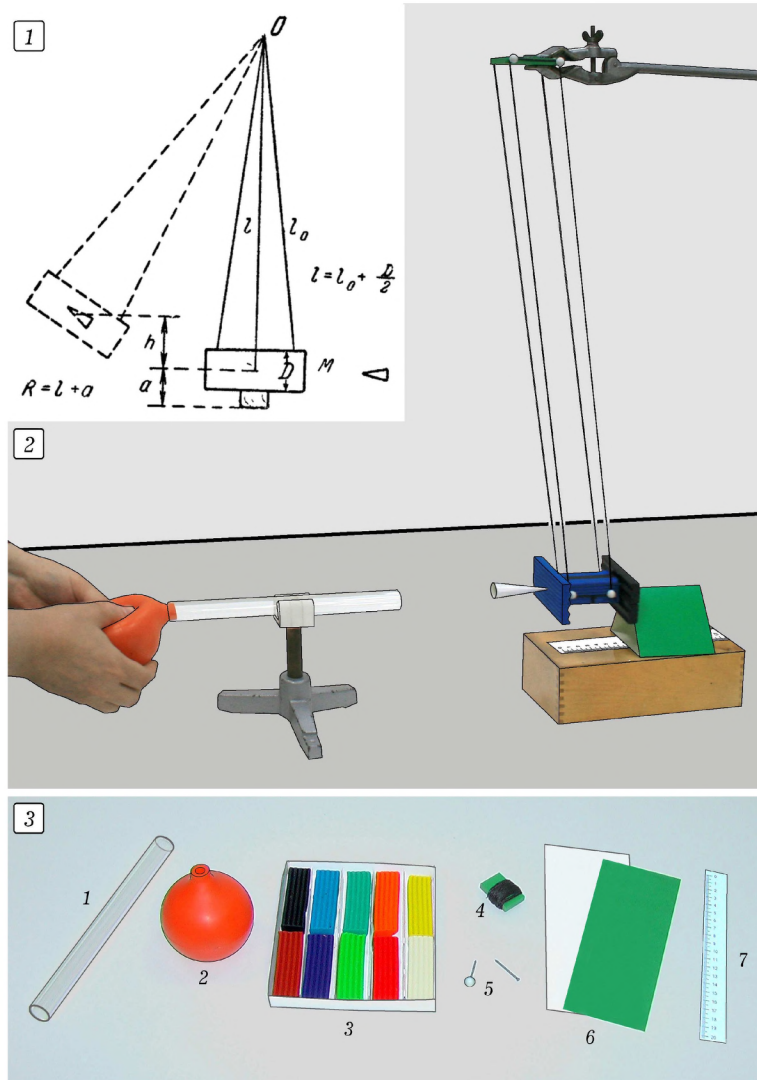
Рис. 3. Совершенствование лабораторного эксперимента по измерению скорости снаряда методом баллистического маятника: 1 — иллюстрация из физического практикума [20, с. 129]; 2 — установка для школьной лабораторной работы (конструкция маятника взята из Интернет-ресурса [22]); 3 — оборудование для организации проектной деятельности школьников по учебному исследованию баллистического метода определения скорости снаряда [23]
