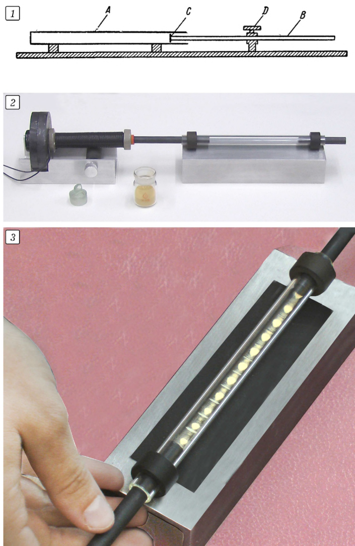
Рис. 4. Совершенствование лабораторного эксперимента по определению скорости звука в упругих средах [20, с. 176–178]: 1 — схема экспериментальной установки университетского уровня [20, с. 177]; 2 — современная экспериментальная установка для школьного практикума; 3 — практический выход проектной деятельности учащихся по исследованию стоячей ультразвуковой волны в воздухе [24]
